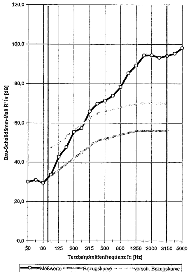
Diagramm: Bau-Schalldämm-Maß R' [dB] Bezugskurve gemäß ÖNORM EN ISO 717-1
